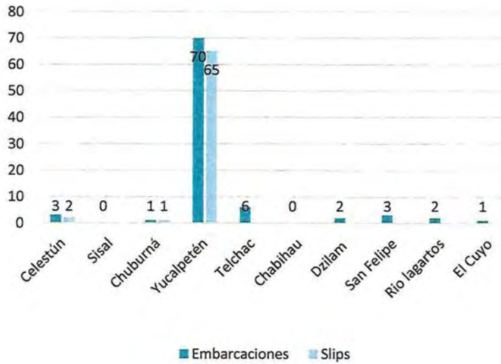
Figura 94 Embarcaciones vs Slips para Embarcaciones Turísticas Mayores a 26"
