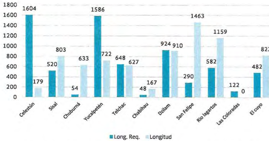
Figura 92 Longitud de ataque vs longitud de ataque requerida para Flota Ribereña
