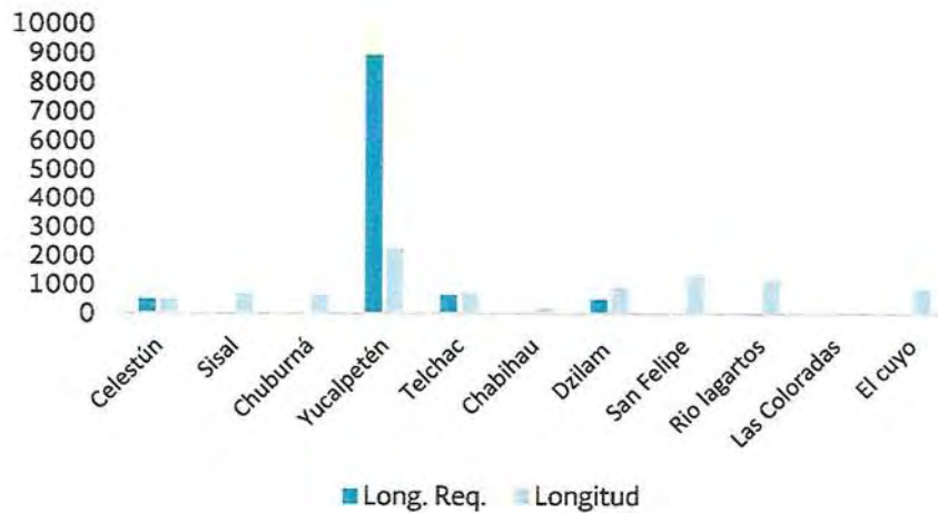
Figura 93 Longitud de Atraca vs Longitud de Atraca requerida para Flota Mayor
